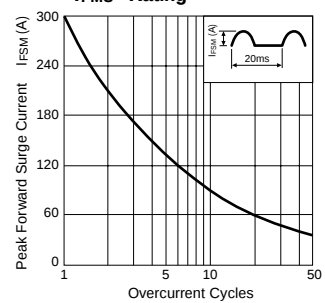
I_{FMS} Rating
